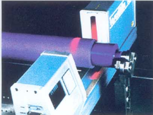
Berührungslose Walzenvermessung
