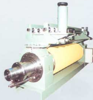
BFI/Sundwig - Planheitsmeßrolle mit MITEX Hochleistungsbeschichtung HIGH DYNAMIC
