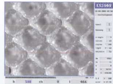
Lasergrafierte 70 Shore D Walzenoberfläche
